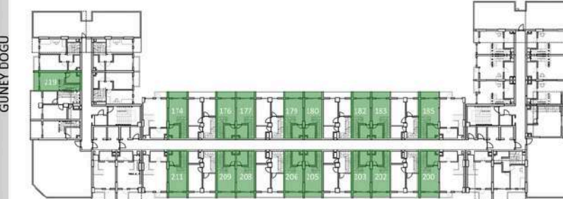
ÇATI KATI PLANI
